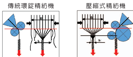
壓縮式紡紗的原理
